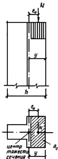
Рис. 5. Внецентренное сжатие
