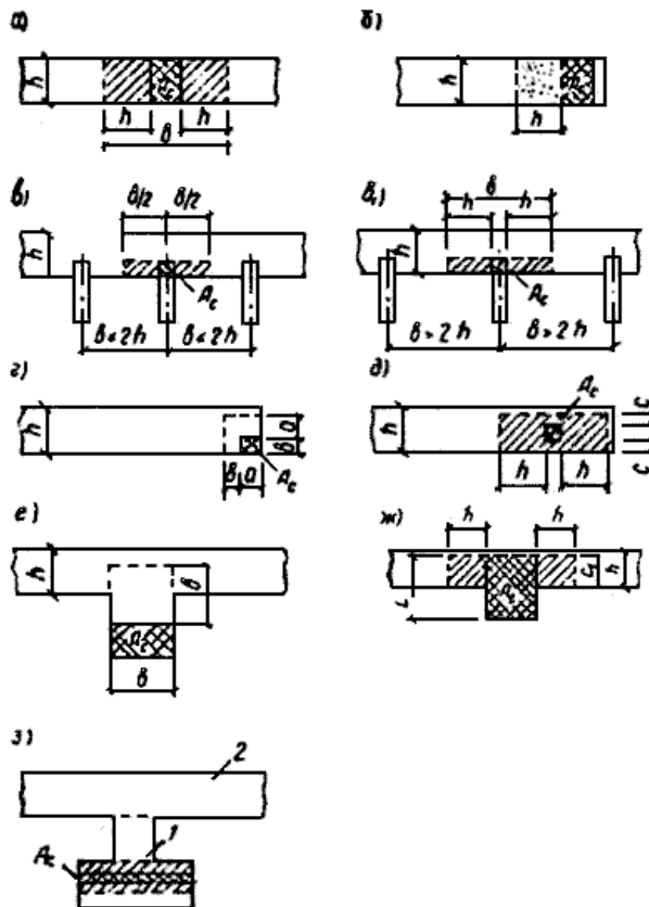
Рис.9. Определение расчетных площадей сечений при местном сжатии
