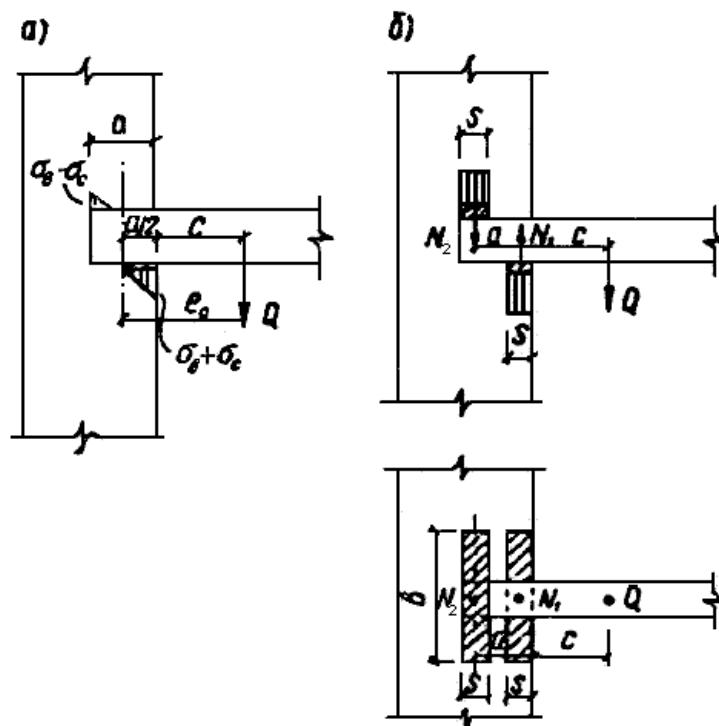
Рис. 14. Расчетные схемы заделки консольных балок
