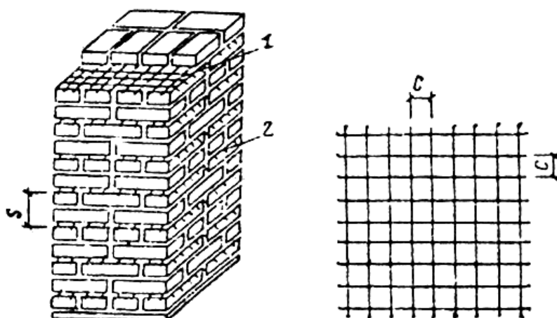
Рис.10. Поперечное (сетчатое) армирование каменных конструкций
